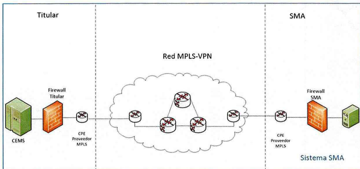
Figura 1: Diagrama de conexión Directa
