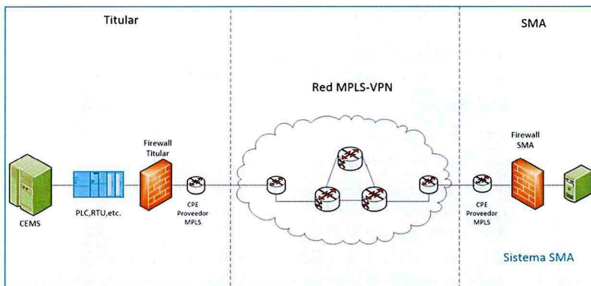
Figura 2: Diagrama de conexión con PLC Espejo
